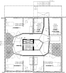
TWEDE VERDIEPING
