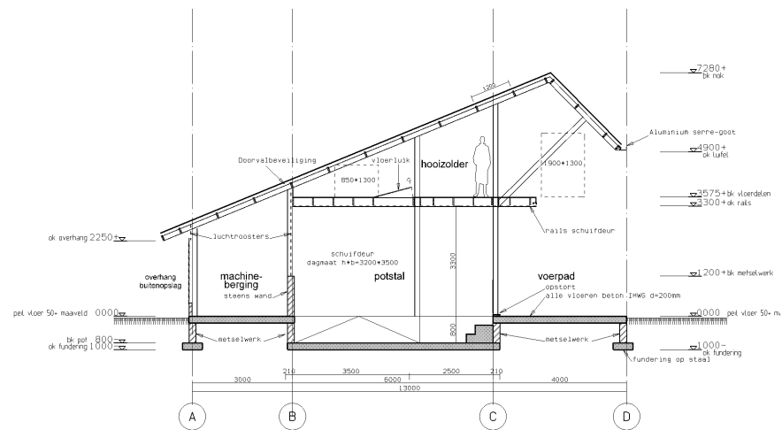
doorsnede AA tussen as 1 en 5
