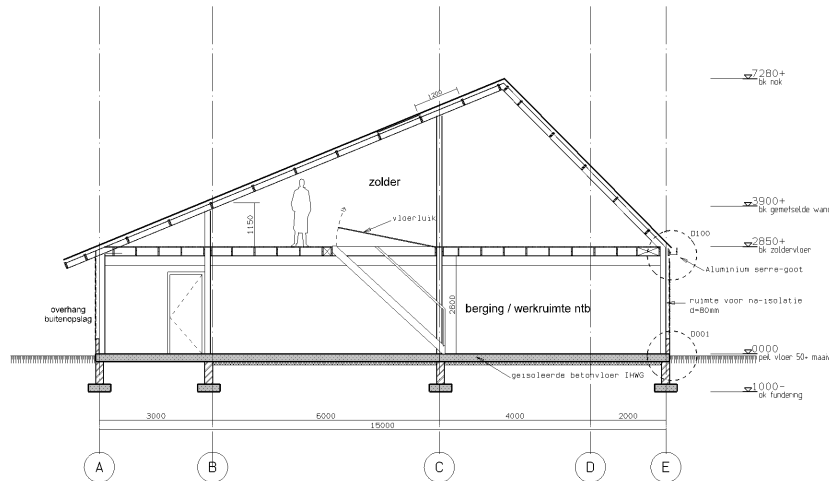
doorsnede CC tussen as 5 en 7
